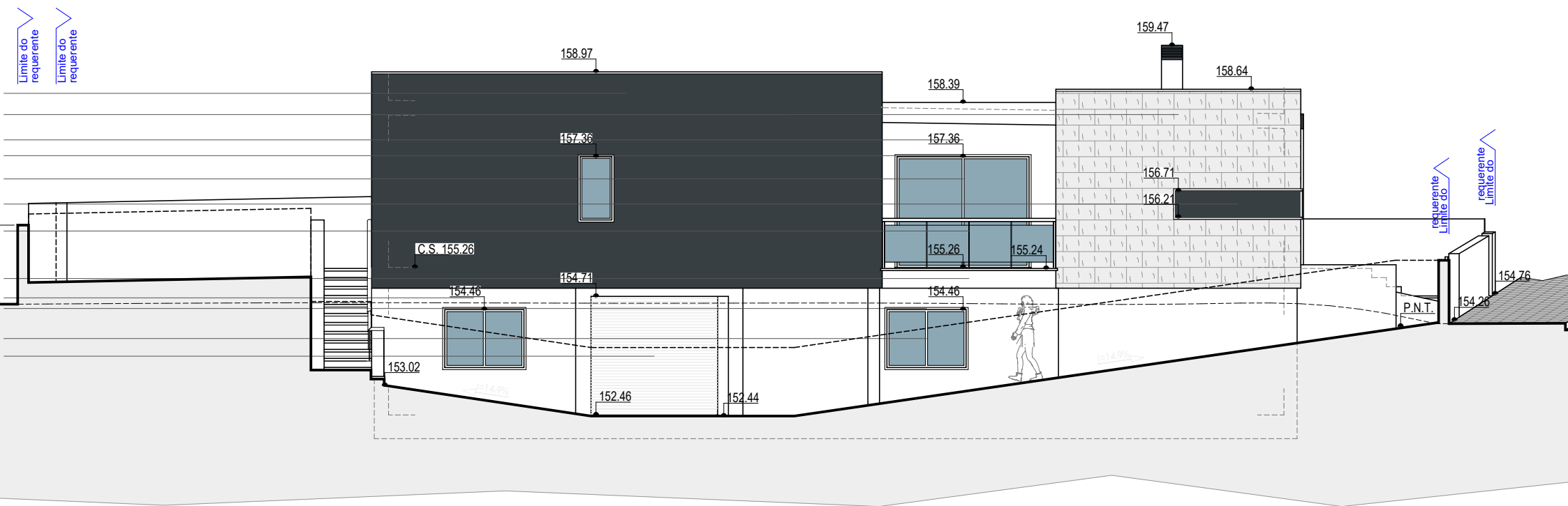
Alçado Lateral Esquerdo
