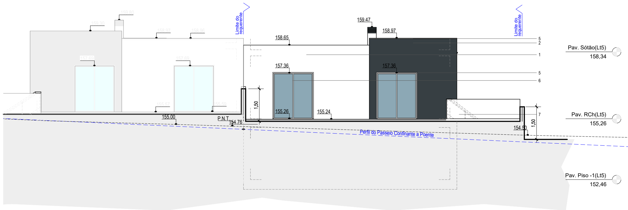
Alçado Posterior
